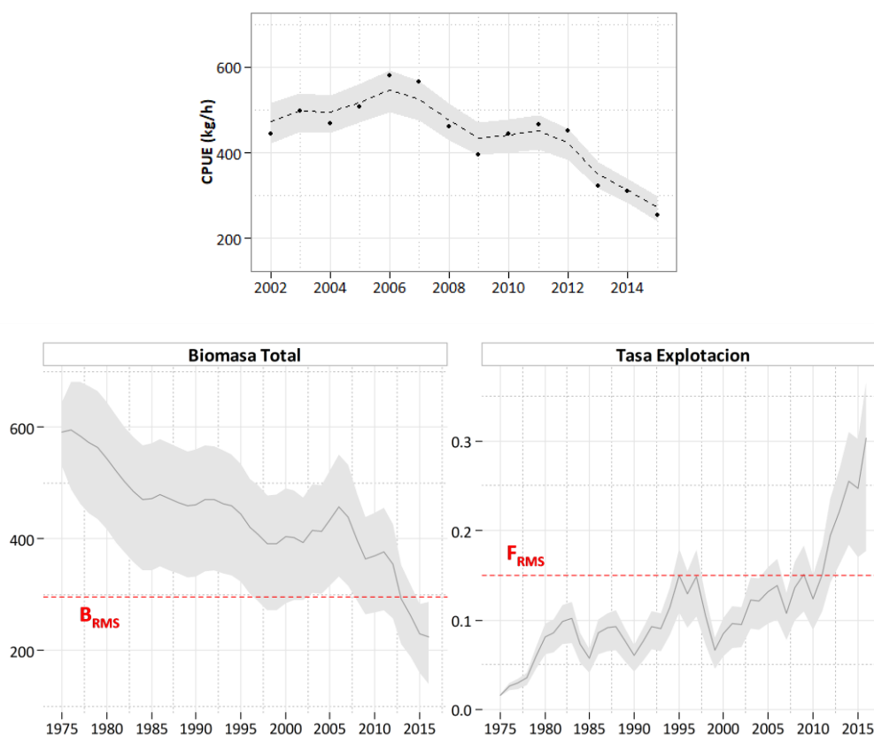
Figura 10. Ajuste del modelo de Schaefer a los datos de CPUE (kg/h), tendencia de la biomasa total (miles de toneladas) y tasa de explotación. La banda sombreada indica el intervalo de probabilidad del 95%. Las líneas horizontales indican la B_{MRS} (295.500 t) y F_{MRS} (0,15).
