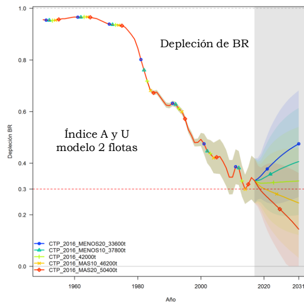
Figura 13. Proyección a captura constante de la depleción de biomasa reproductiva con la incertidumbre asociada para cada uno de los índices y de los escenarios de captura considerados.
