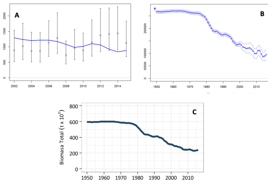
Figura 11. (A) Resultados del ajuste del índice A-U, (B) trayectorias de biomasa reproductiva y (C) biomasa total a partir de la aplicación del modelo estructurado por edades.
