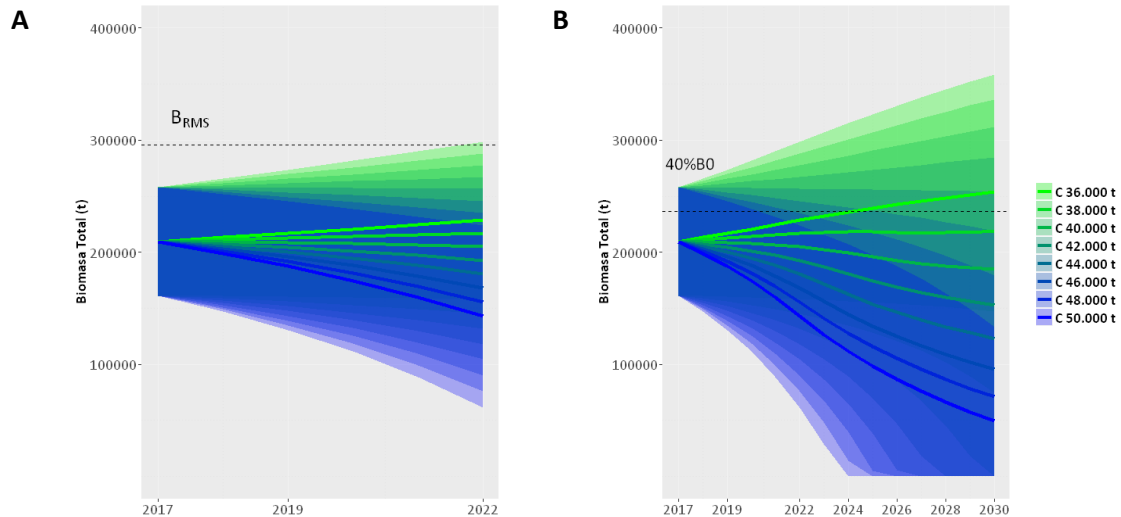
Figura 12. Proyecciones del modelo global para la biomasa total de corvina en diferentes escenarios de capturas constantes. A) PBR = B_{RMS} B) PBR = 40\% B_0
